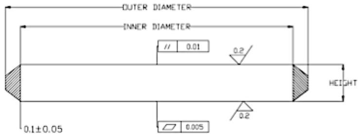
DS TYPE(DOUBLE BLADE, SINGLE BEVEL TYPE)
